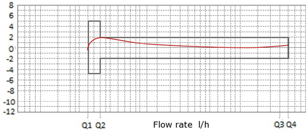
Error %
